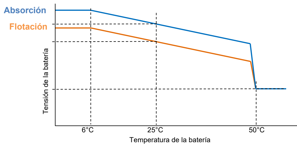
Figura 20 Gráfico de la compensación de temperatura para tensiones de flotación y absorción
