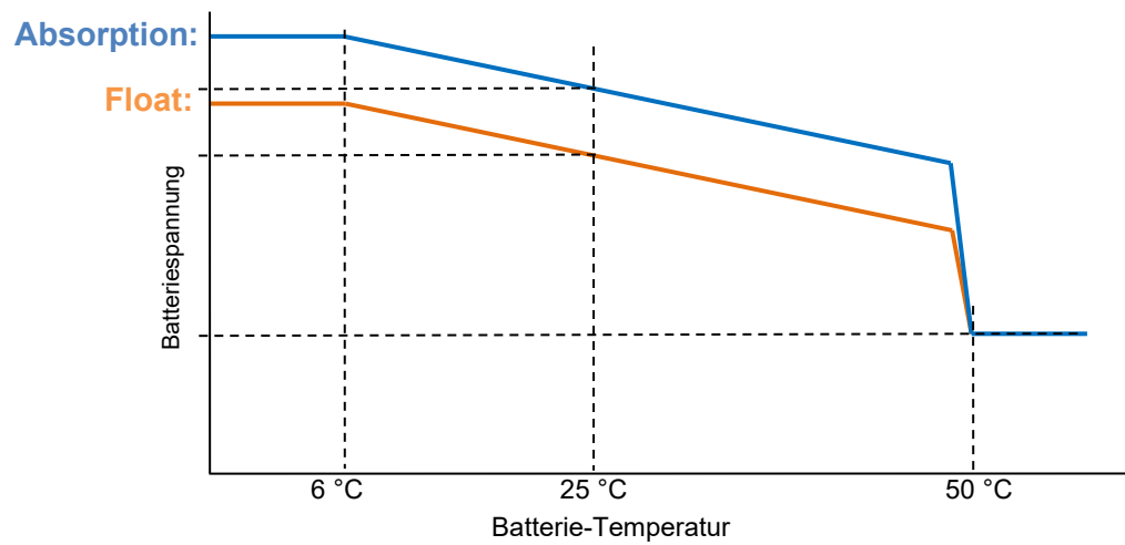
Abbildung 16 Grafik zum Temperaturausgleich für die Spannungswerte der Ladeerhaltungs- und Konstant Spannungs-Phasen
